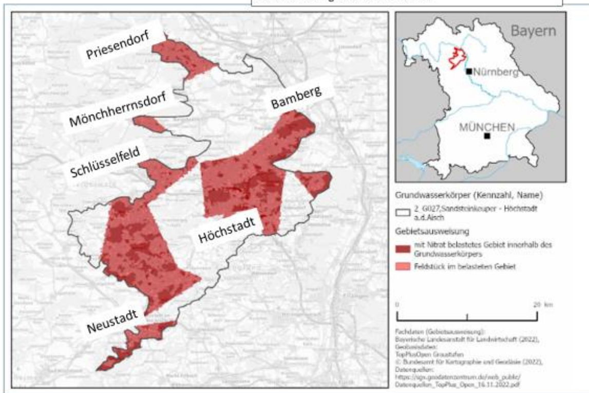
Abb. 1: Mit Nitrat belastete Gebiete und Lage des Grundwasserkörpers
